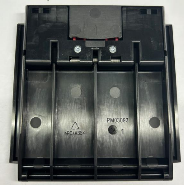
图二，检查组件装配到位后，按压红色按键可回弹顺畅。
