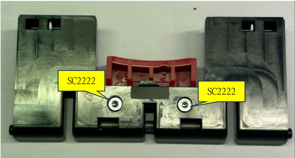
图二，检查图一装配到位后在两孔位锁上 SC2222 螺丝。
