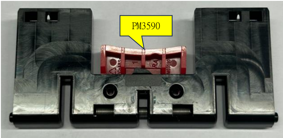
图一，将 PA3581-1 和 PM3590 组装在一起，注意孔位对正
