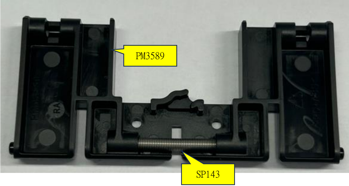
图一，将 SP143 装入 PM3589 两边孔径，注意需装配到位。
