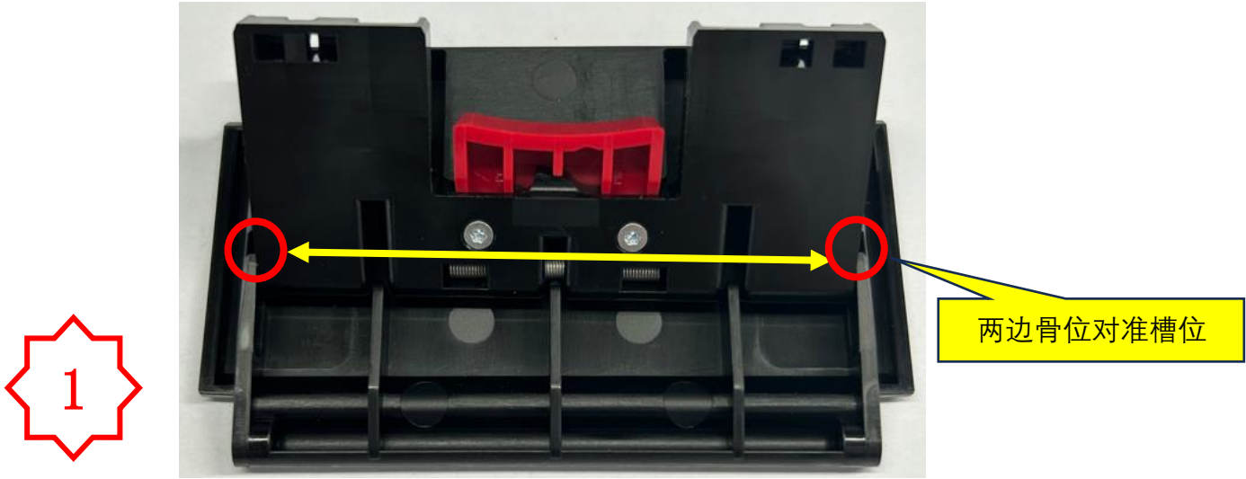
图一，将 PA3581-2 上的 PM3589 两边骨位对准和 PM3092 上的槽位装入，再将红色按键先往弹簧方向按压并装进 PM3092 中间孔位。
